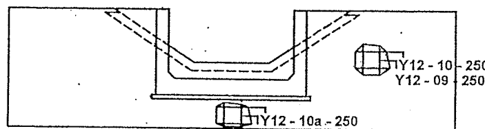
SECTION E - E
