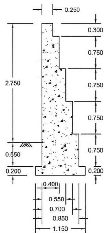
SECTION A-A
