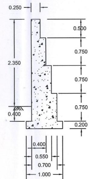
SECTION D-D
